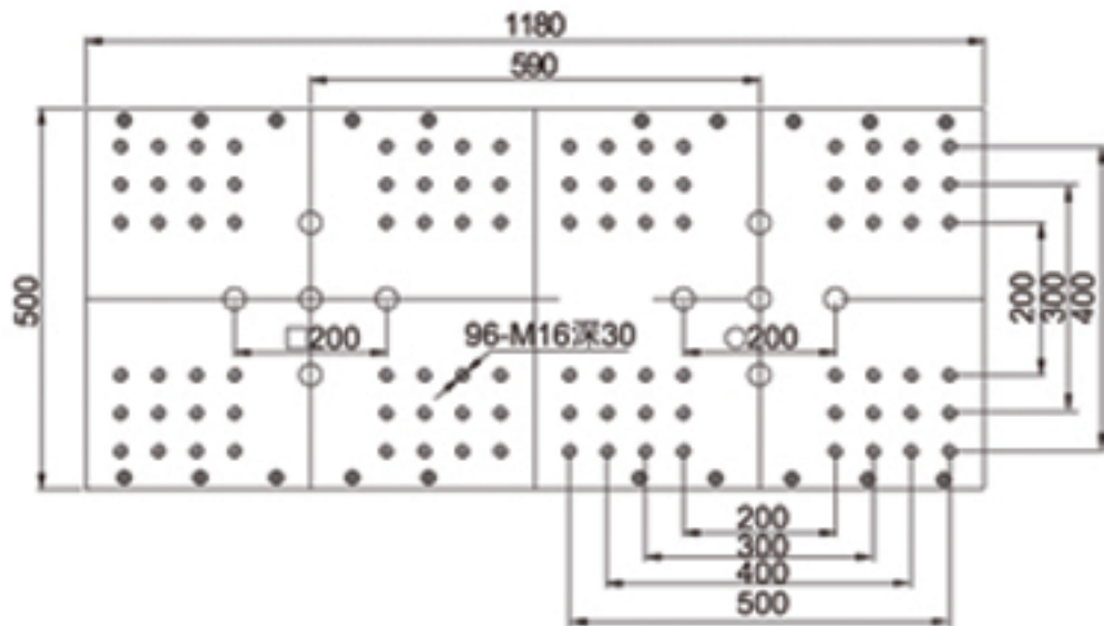
双滑板 / Double Slide
